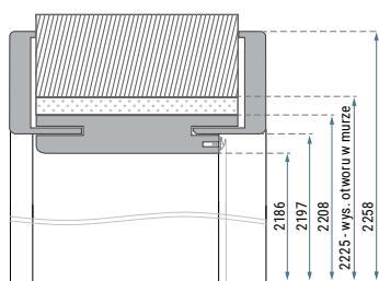
Wymiary ościeżnicy do drzwi PN22.
