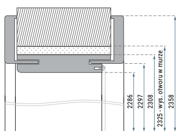
Wymiary ościeżnicy do drzwi PN23.
