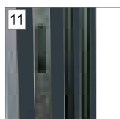
Przegroda termiczna, dwie uszczelki w ościeżnicy
