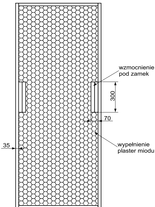
Budowa skrzydła płytowego
