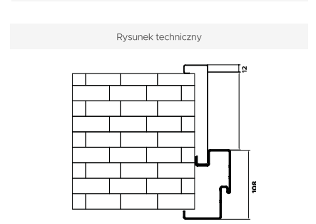
Portal z ościeżnicą wewnętrzną Iron
