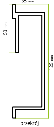
przekrój
