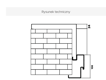
Portal z ościeżnicą regulowaną Iron
