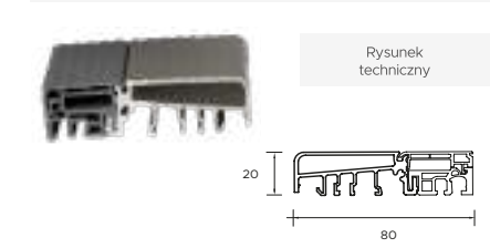
Ciepły próg PVC/ALU z przegrodą termiczną Prestige, Optimum
