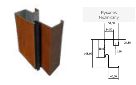
Próg aluminiowy Optimum,
