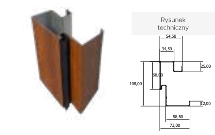
Ciepły próg PVC/ALU z przegrodą termiczną Prestige, Optimum
