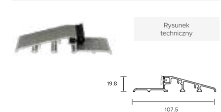
Próg aluminiowy z uszczelką Premium, Normal, Protect, Iron do ościeżnicy "9" (kątovej), "11" (wewnętrznej)
