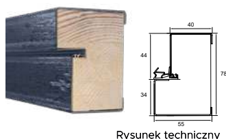
Ciepły próg PVC/ALU z przegrodą termiczną Alu Hybrid
