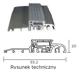
Próg aluminiowy Optimum, Prima
