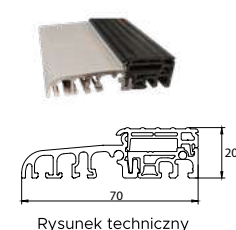
Próg ciepły ALU i PVC Prima
