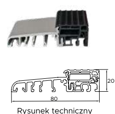
Trwały próg ze stali nierdzew- nej z uszczelką do Basic 3.0
