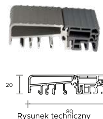
Ciepły próg PVC/ALU z przegrodą termiczną do Plus
