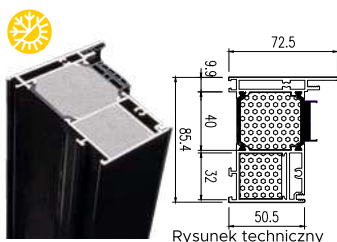
Próg ze spadkiem Optimum, Termo Prestige Lux
