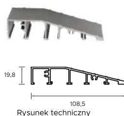
Próg aluminiowy Optimum, Prima
