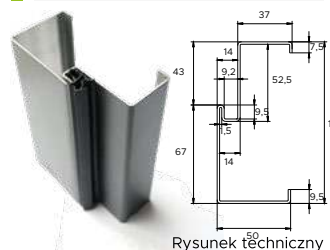
Przekrój łącznika kąto- wego Termo 90°
