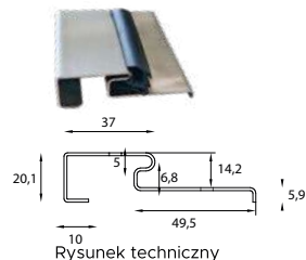
Trwały próg ze stali nierdzew- nej z uszczelką do Basic 3.0
