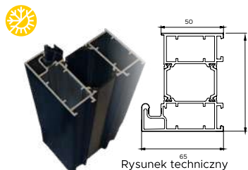
Ościeżnica kątowa Prima
