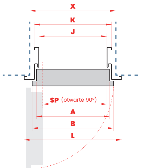
PRZĘKÓJ POZIOMY
