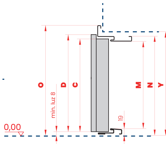
PRZĘKÓJ PIONOWY
