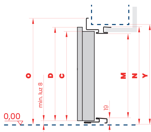
PRZEKRÓJ PIONOWY
