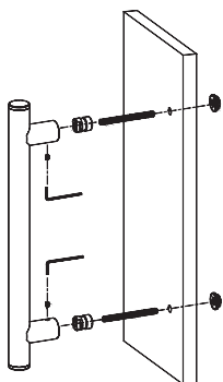
MONTAŻ POCHWYTU JEDNOSTRONNEGO NA PRZESTRZAŁ
