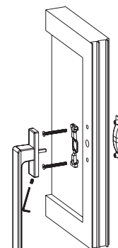
MONTAŻ KLAMKI OKIENNEJ I BALKONOWEJ
