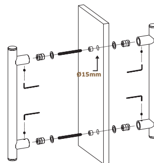
MONTAŻ POCHWYTU DWUSTRONNEGO DO DRZWI SZKŁANYCH
