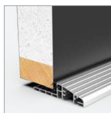
3 przylgi skrzydła
