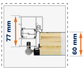
Ościeznica ALUTHERM 60*
