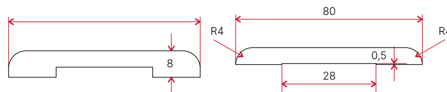
Przekrój opaski maskującej
