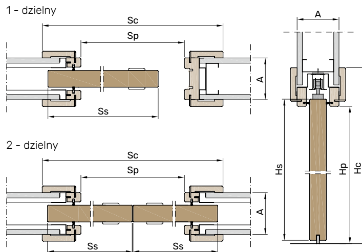
System wewnątrzścienny
