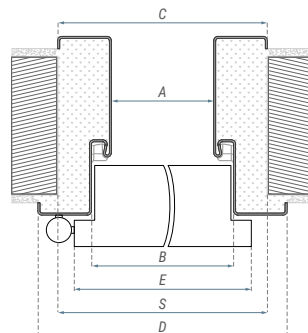
Wymiary ościeżnicy stalowej stałej PPOŻ [mm]
