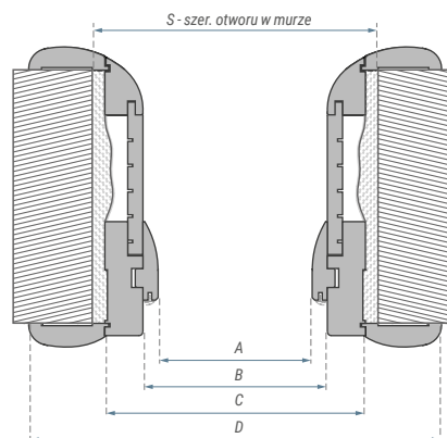
Wymiary ościeżnicy New Arcus [mm]:
