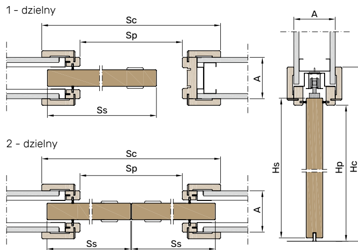
System wewnątrzścienny
