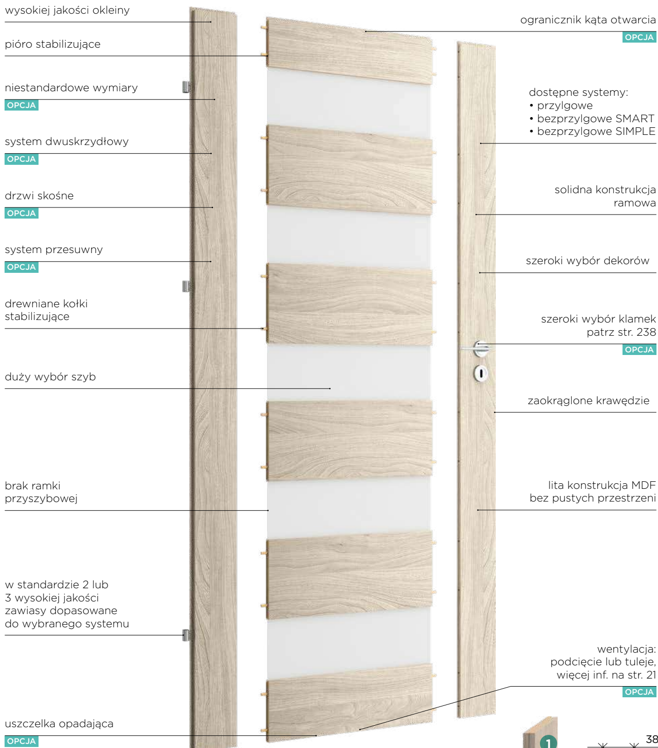
Konstrukcja ramowa
