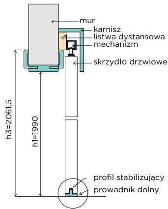
OPASKA 60 mm H1 = 1990 mm
