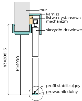
OPASKA 80 mm H1=1990 mm
